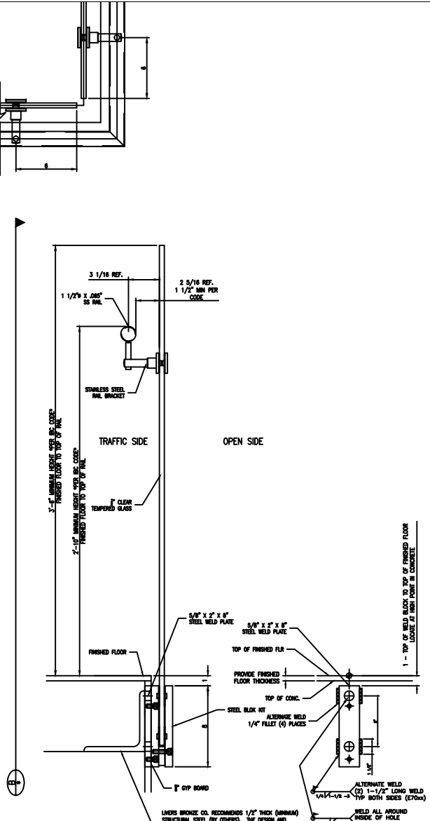
SECTION SCALE: 3" = 1'-0"
