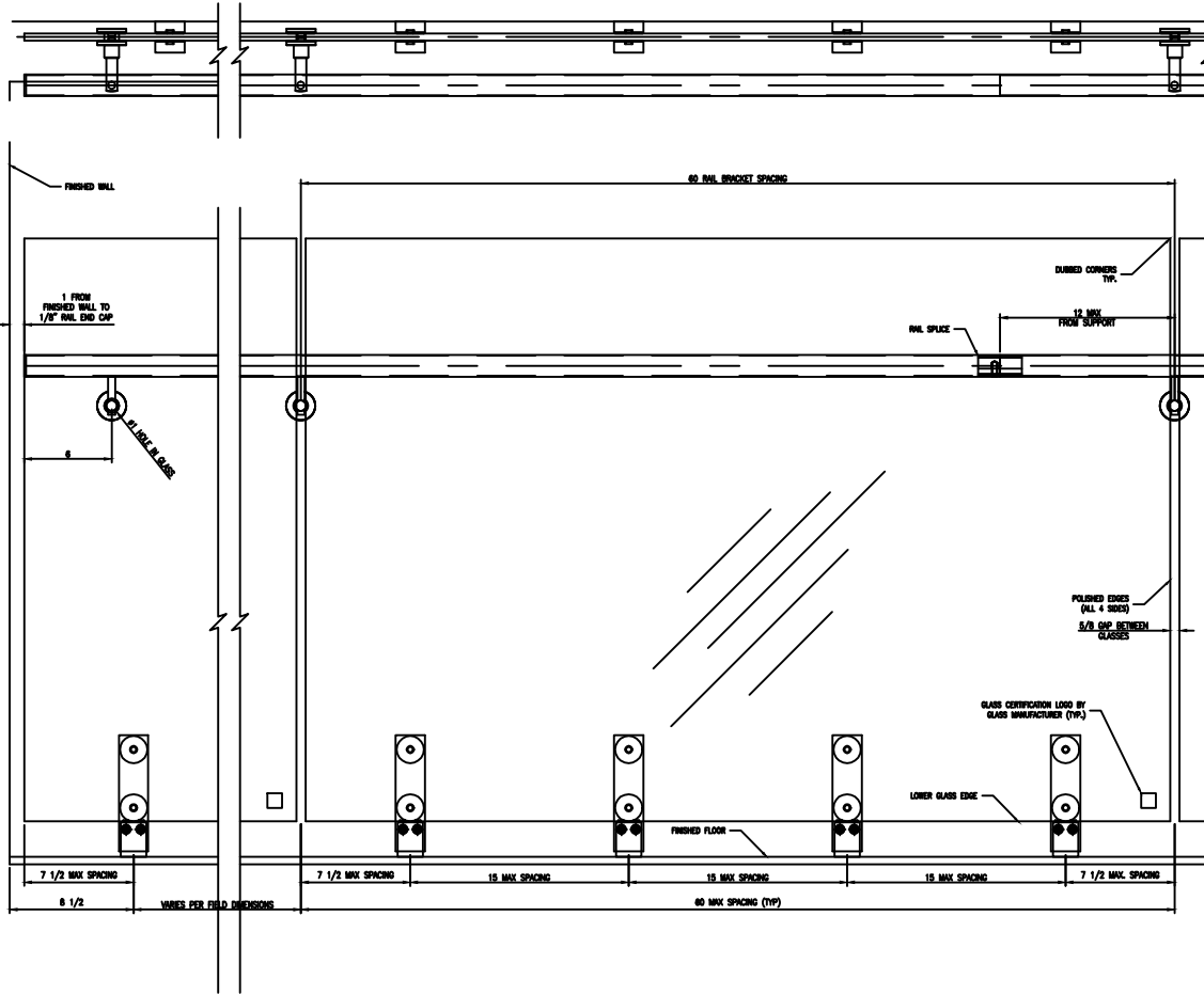
B ELEVATION SCALE: 3" = 1'-0"
