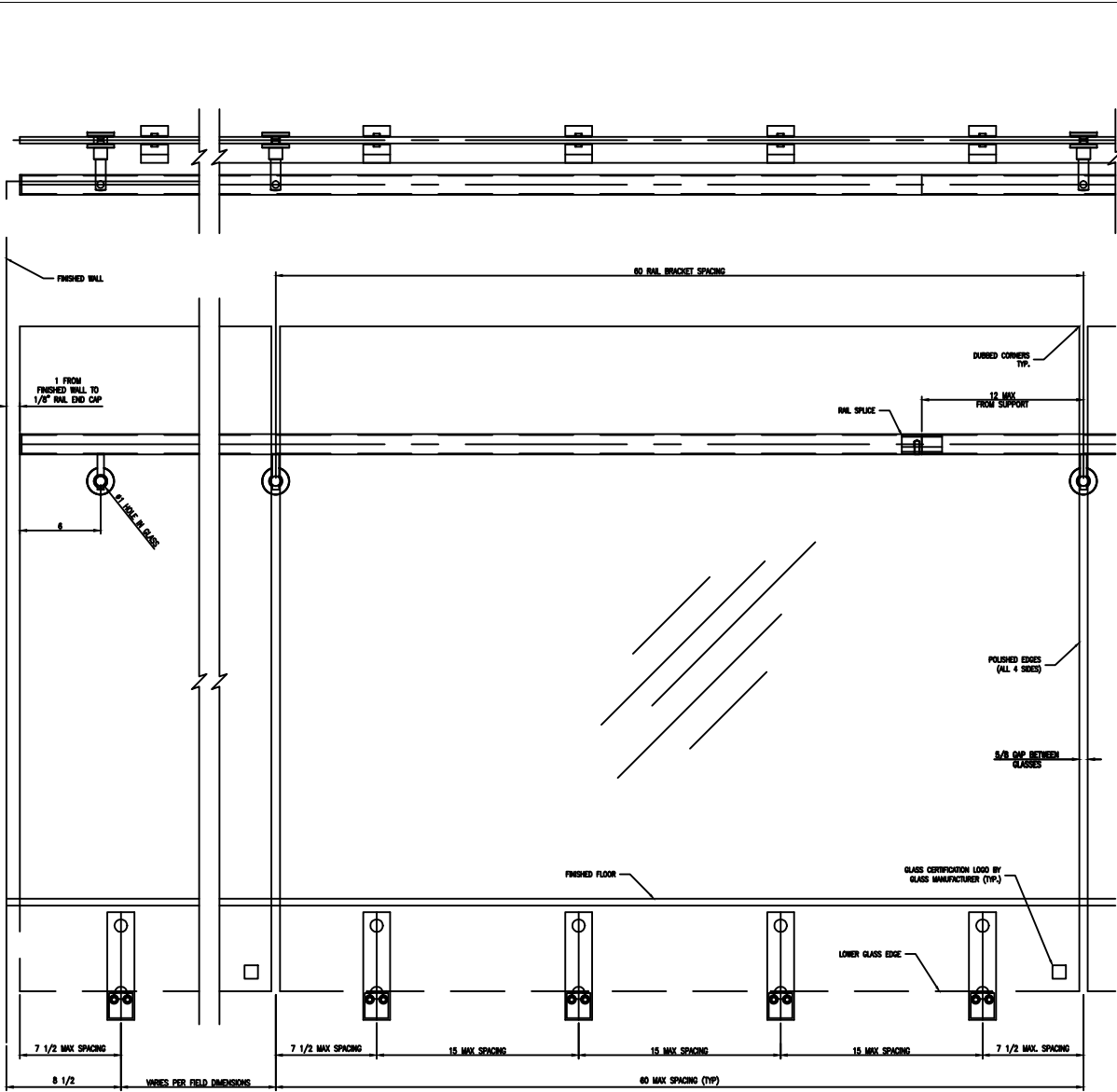
ELEVATION SCALE: 3" = 1'-0"
