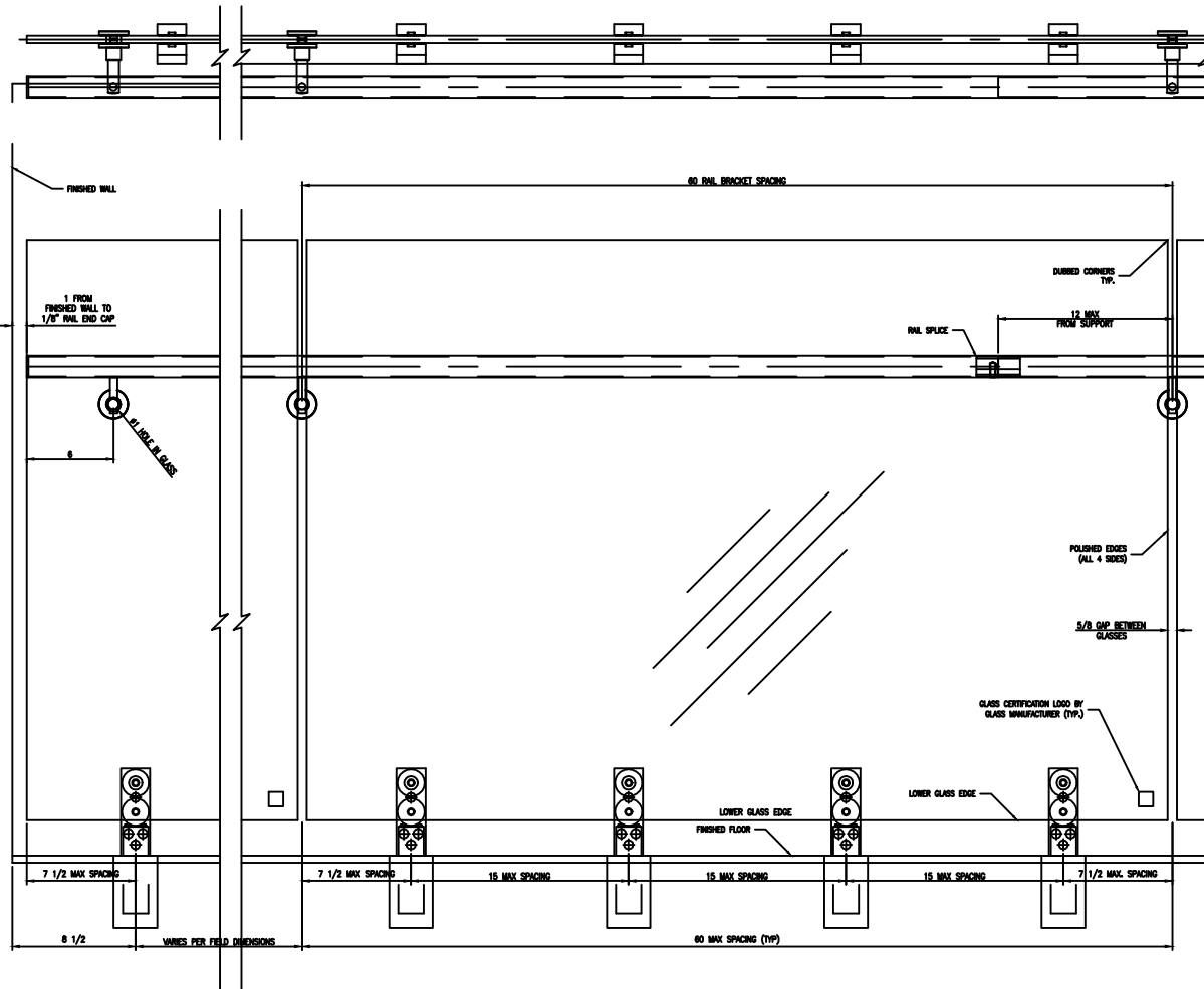
B ELEVATION SCALE: 3" = 1'-0"
